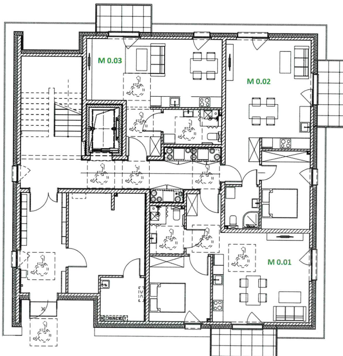
RZUT PARTERU
