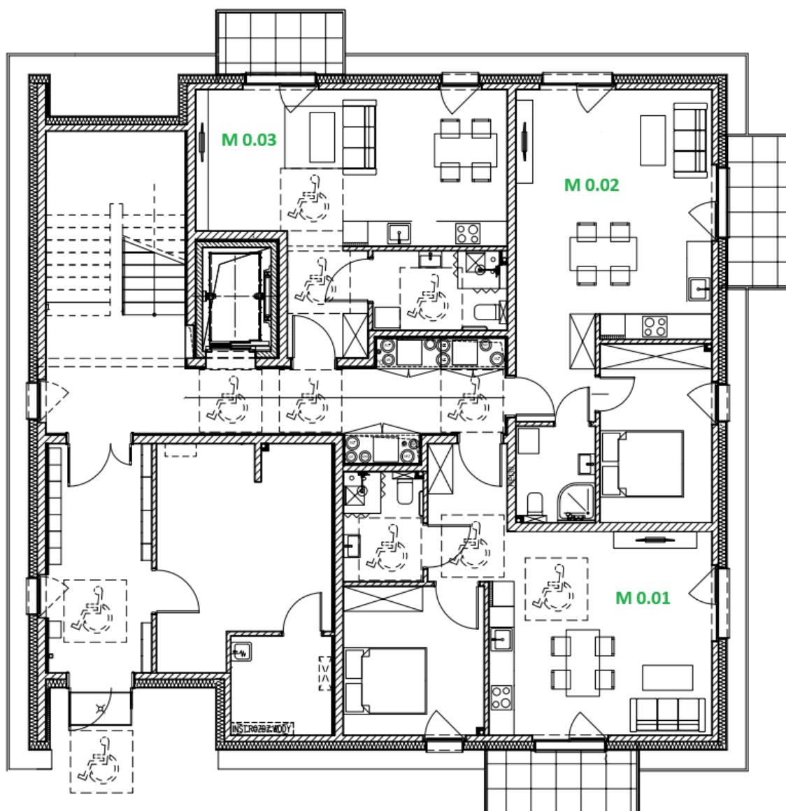
RZUT PARTERU
